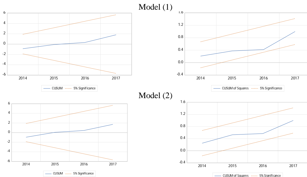
الشكل رقم (2): اختبارات الاستقرار الهيكلي CUSUM , CUSUM of squares
